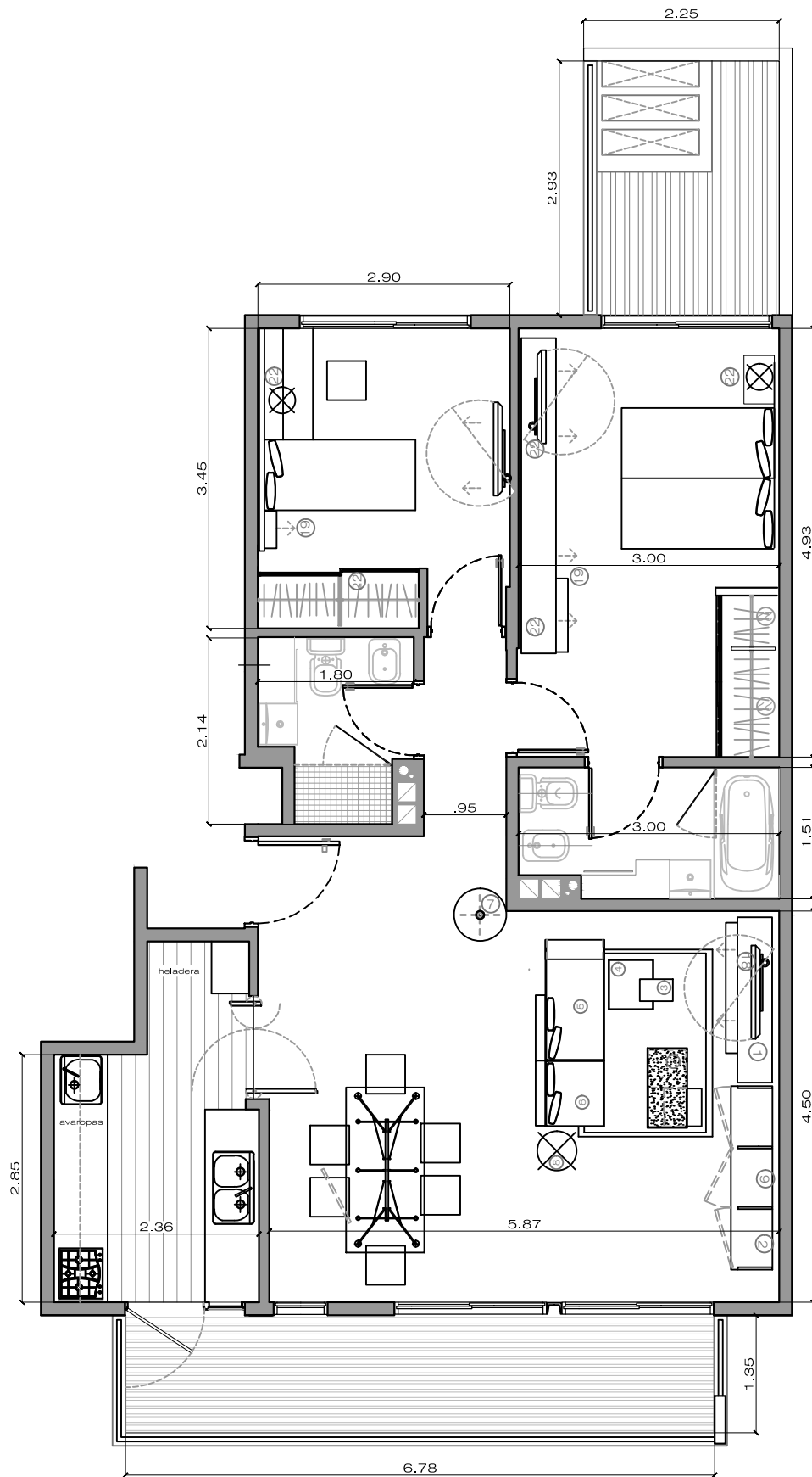
Depto B 1º PISO
